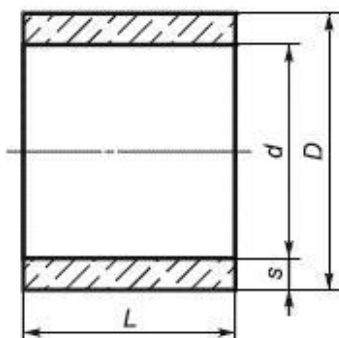
Рисунок 2 - Безнапорная муфта
