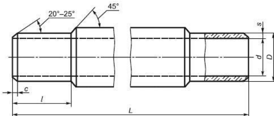
Рисунок 3 - Напорная труба
