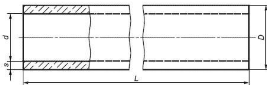
Рисунок 1 - Безнапорная труба
